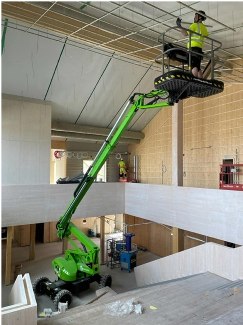
Pågående montage av undertak i Stora Hjärtat
